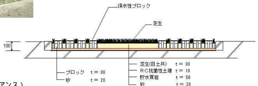
断面詳細図
